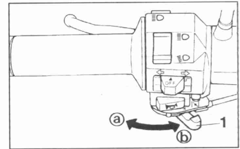
1. Palanca del estrangulador (choke) “|X|”
