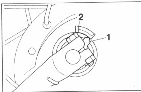
1. Indicador de desgaste 2. Línea del límite de desgaste
